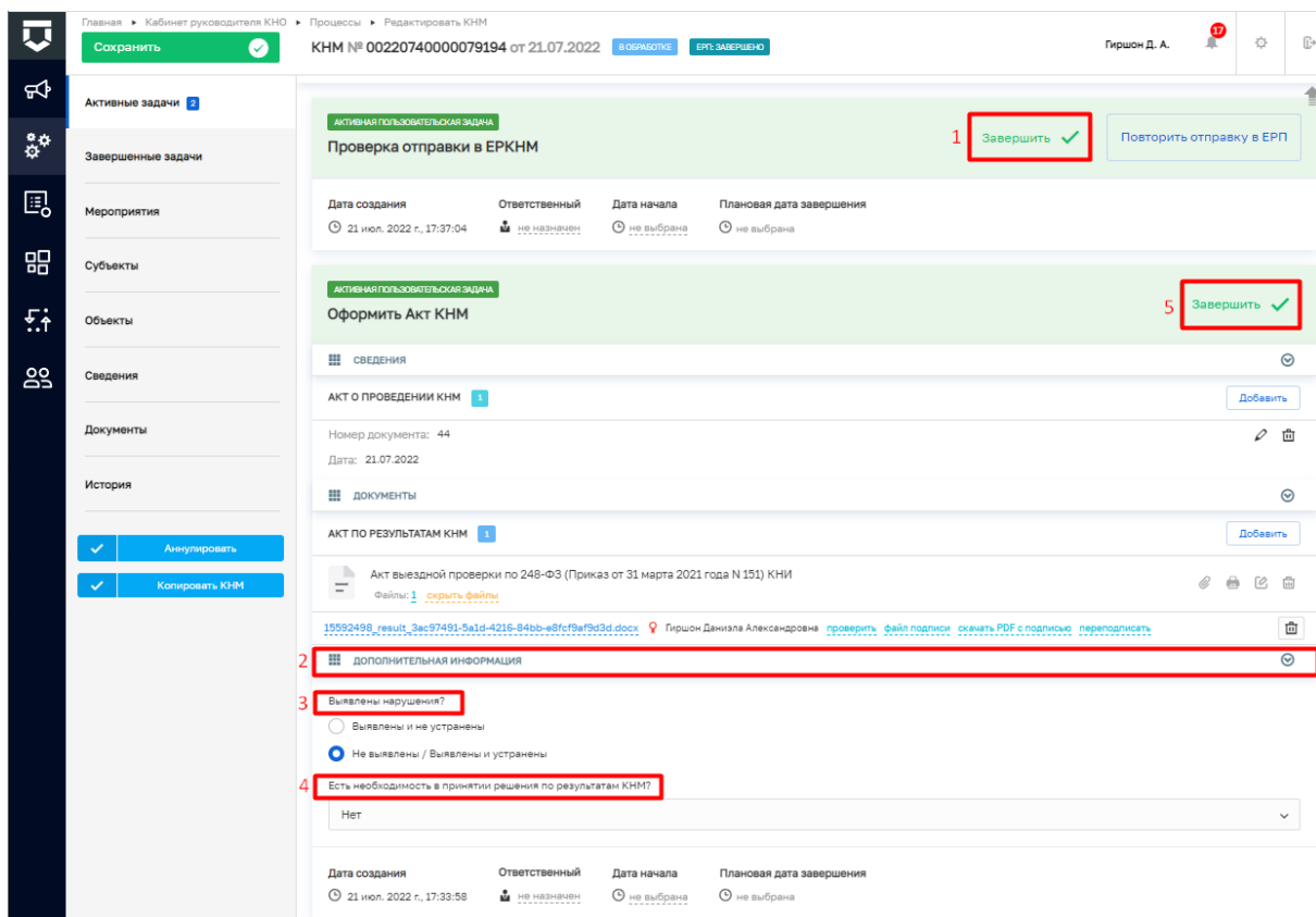
Рисунок 35. Работа с задачами "Проверка отправки в ЕРКНМ" и "Оформить Акт КНМ"
